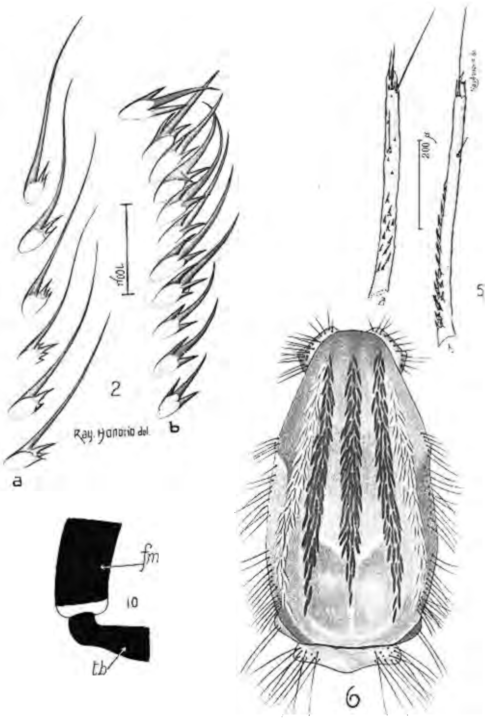
Fig. 2—♀ Psorophora genu-maculata . Escamas do pecten do siphão respiratório (a) e escamas do VIII segmento abdominal (b) da larva. Original.
